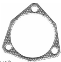
Junta de saída do escape S-10 Motor MUM Sprint 4.07 sem anel
